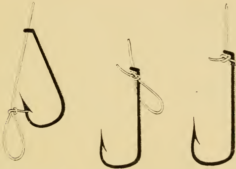
Fig. 80. Befestigen geührter Angelhaken an der Schnur durch den Galeerenknoten
