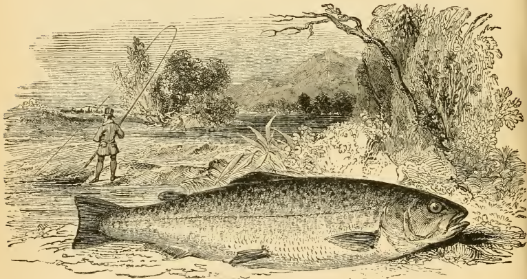
Fig. 320. Bachforelle.
